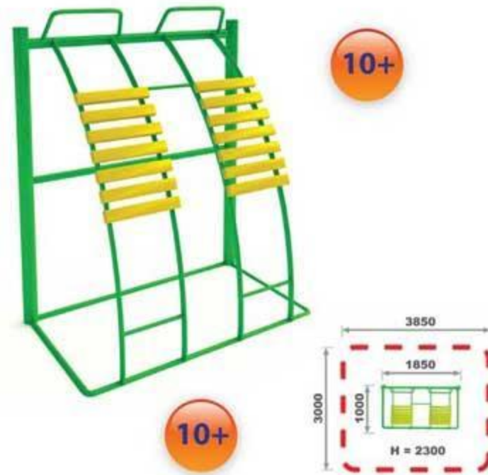
тренажер "Верхняя тяга" CO-3 1 62 00
