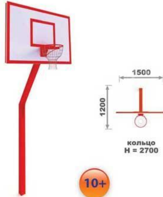
СП-1.31 "Баскетбольная стойка"
