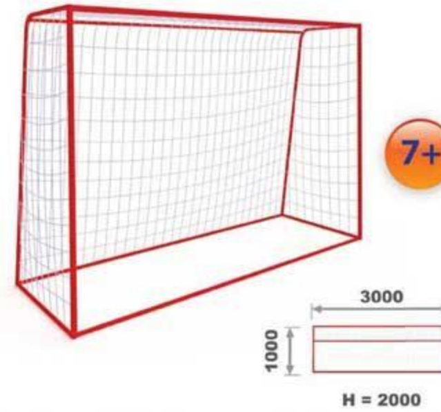
СП-1.56 "Ворота для мини футбола"
