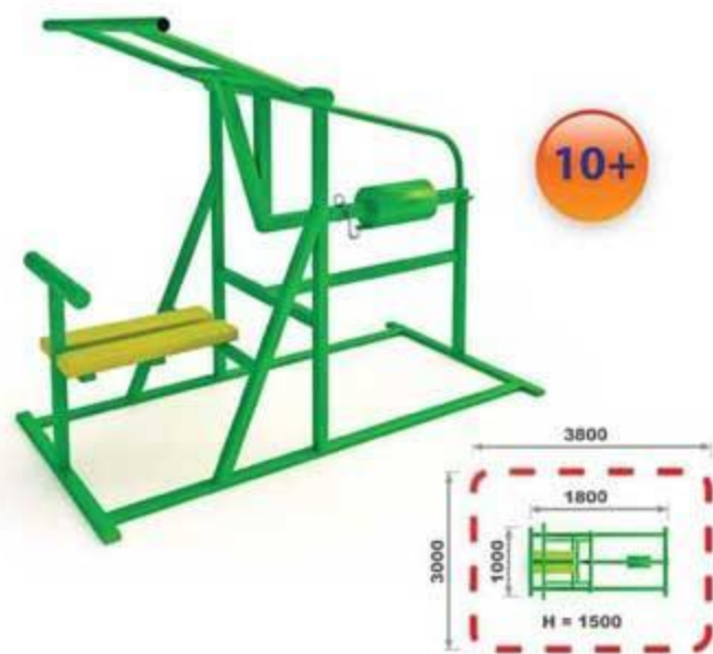
СП-1.42 "Стальной пресс"
